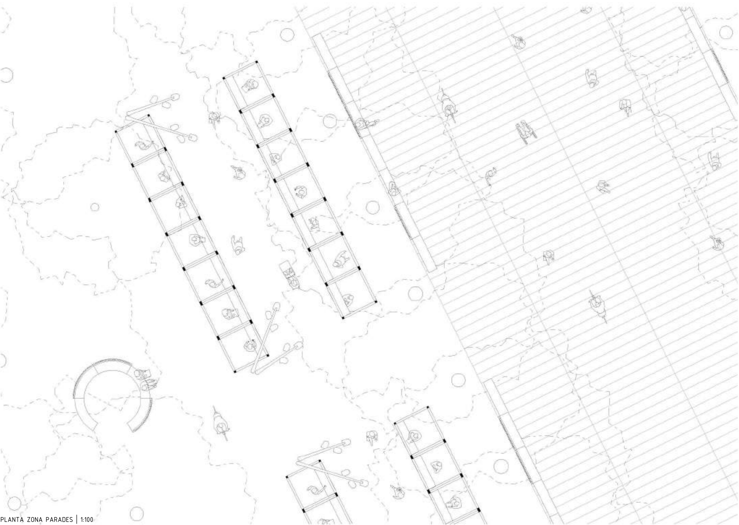
PLANTA ZONA PARADES | 1:100
