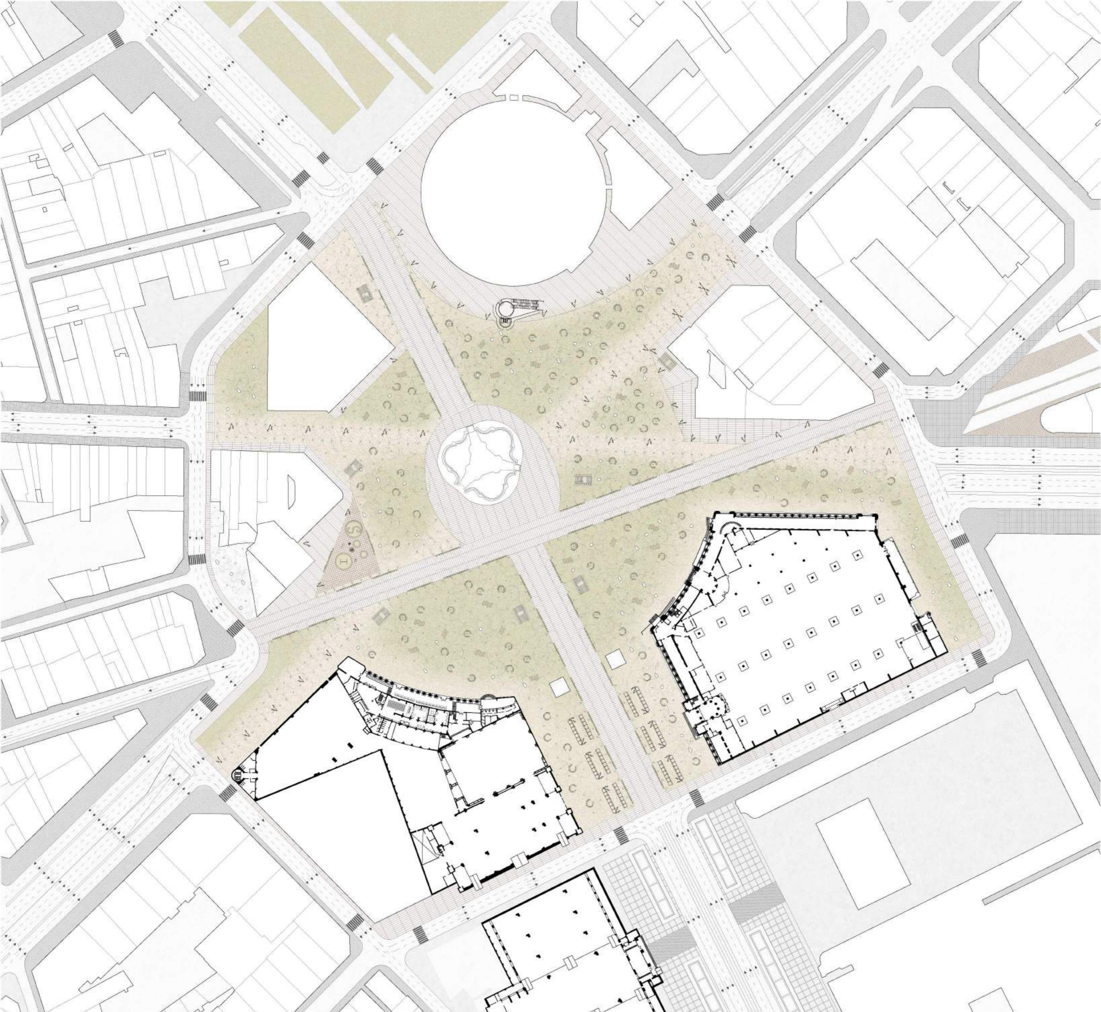
PLANTA PAVIMENTS | 1:1000
